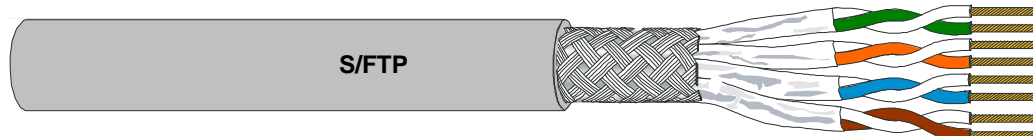
Gesamtschirm: Kupfergeflecht Paarschirmung: Alufolie
